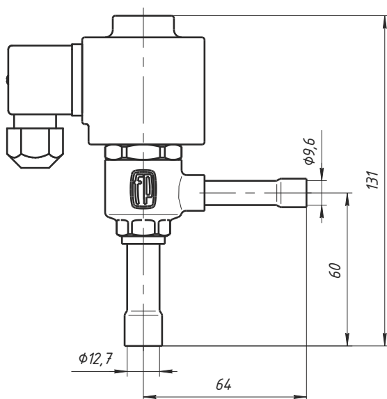
Рис. 4. Габаритные и присоединительные размеры
