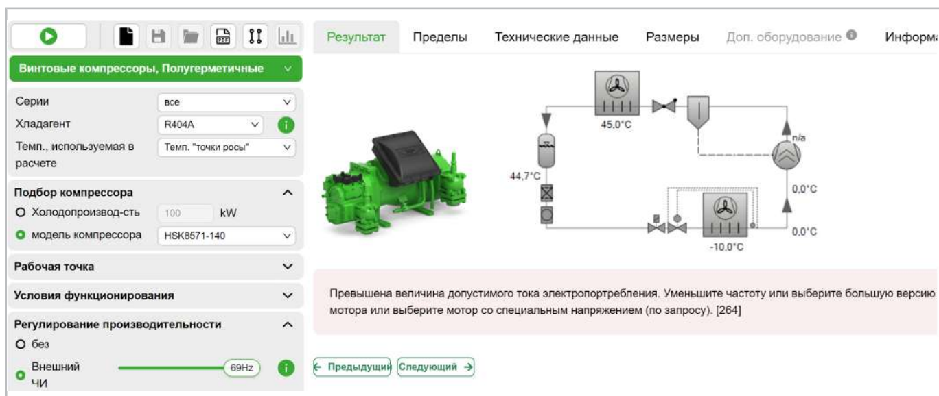
Рис. 8: Увеличивая рабочую частоту выбранного компрессора, можно превысить максимальное потребление тока. В этом случае программа рекомендует более мощную версию мотора или мотор со специальным напряжением.
