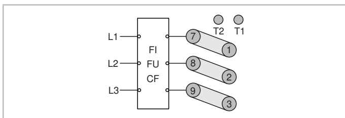
Abb. 14: Motoranschlüsse an der Stromdurchführungsplatte bei Betrieb mit externem Frequenzumrichter (FU) für Schraubenverdichter
