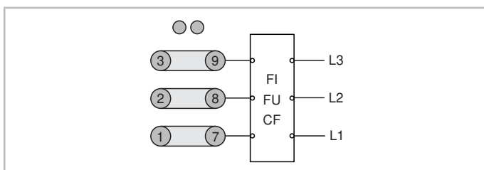
Abb. 16: Motoranschlüsse an der Stromdurchführungsplatte bei Betrieb mit externem Frequenzumrichter (FU) für Schraubenverdichter HS.53
