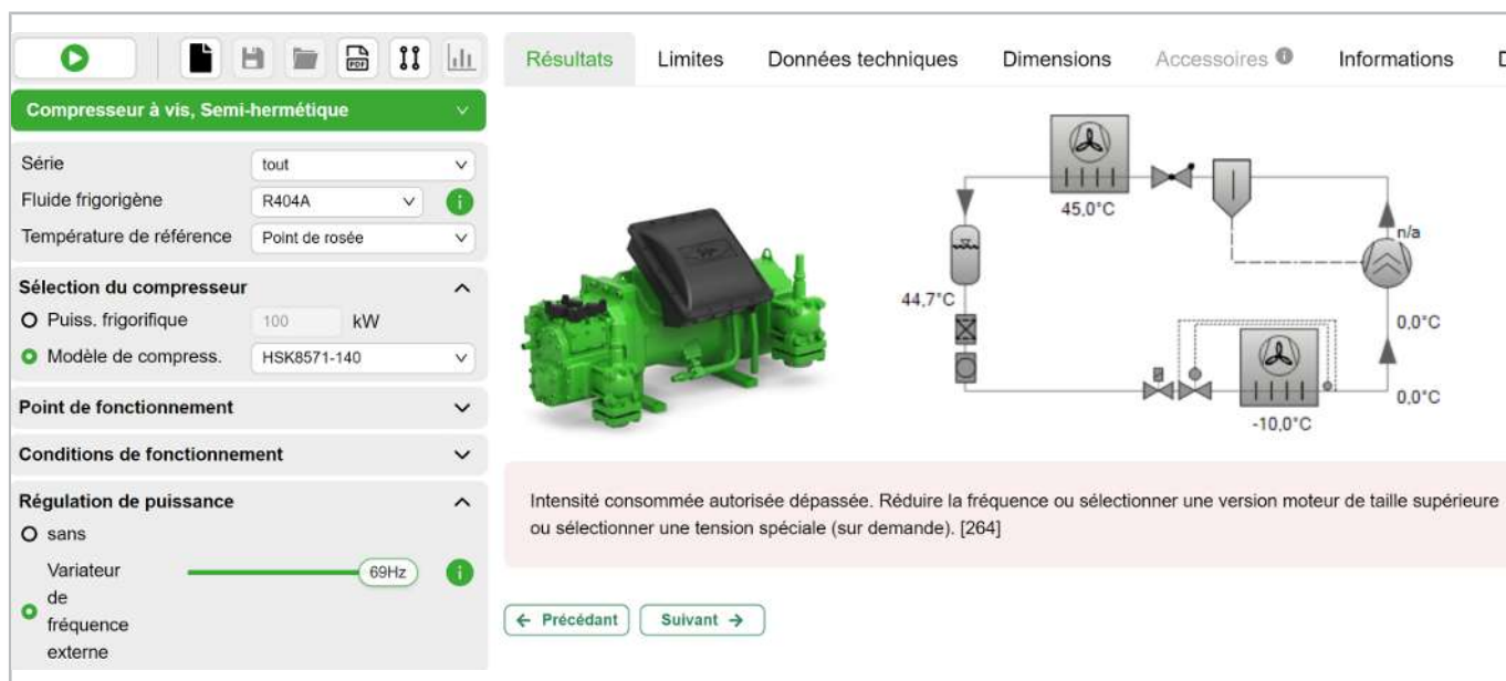
Fig. 8: Si la fréquence de service d'un compresseur sélectionné est augmentée, le courant absorbé maximal peut être dépassé. Dans ce cas, le logiciel recommande l'utilisation d'une version de moteur plus grande ou un moteur à tension spéciale.
