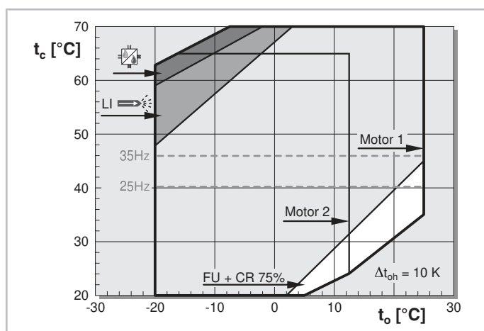
Рис. 6: Пример областей применения для винтовых компрессоров CSH с преобразователем частоты (FI) для хладагента R134a. Компрессор можно эксплуатировать только ниже указанных линий частот.
