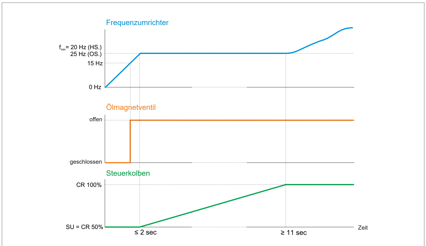
Abb. 21: Empfohlene Anlaufsequenz für Verdichter OS.53 .. 74, HS.53 .. 74 mit Frequenzumrichter (FU). Steuervolben entlastet anfahren, Ölmagnetventil öffnen, sobald der FU 15 Hz erreicht. Bei Erreichen der Mindestdrehzahl (20 Hz für HS., 25 Hz für OS.) Steuervolben zuschalten auf 100% (siehe Betriebsanleitung SB-100 für HS. bzw. SB-500 für OS.).
