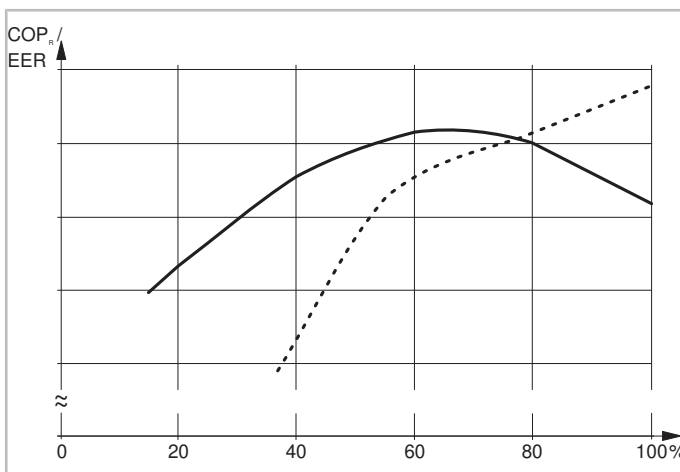
Abb. 2: Vergleich der Leistungsregelungs-Effizienzcharakteristik von Schraubenverdichtern mit Schieberregelung vs. Frequenzumrichter (FU): Leistungszahl COP_r/EER (Verhältnis Kälteleistung zu aufgenommener Leistung) in Abhängigkeit von der Last.
