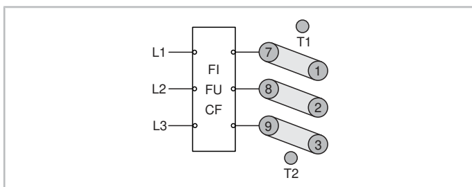
Abb. 15: Motoranschlüsse an der Stromdurchführungsplatte bei Betrieb mit externem Frequenzumrichter (FU) für Schraubenverdichter HS.64 ..
