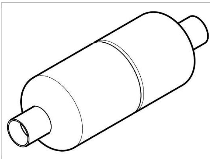
Abb. 28: Einfacher Pulsationsdämpfer SD42 im ECO-Anschluss, Teilenr. 354 004 05
