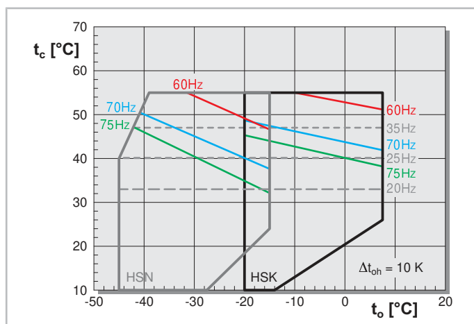
Fig. 5: Exemple des limites d'application du compresseur à vis HS.64 avec convertisseur de fréquences et fluide frigorigène R404A. Le compresseur ne peut être utilisé que dans la plage au-dessous des lignes de fréquence indiquées.
