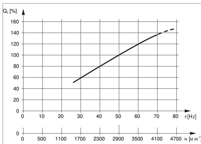
Fig. 4: Évolution typique de la puissance frigorifique Q_0 en fonction de la vitesse de rotation et de la fréquence pour les compresseurs à vis
