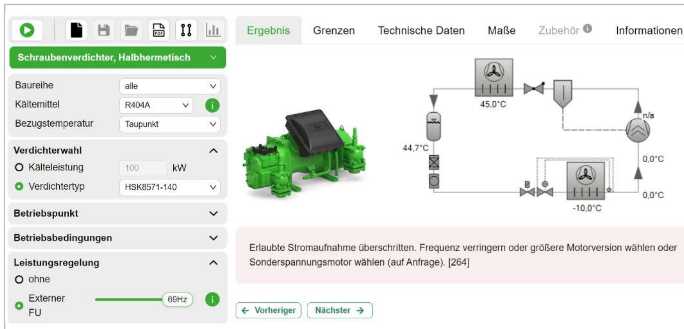
Abb. 8: Erhöht man die Betriebsfrequenz eines gewählten Verdichters, kann die maximale Stromaufnahme überschritten werden. Die Software empfiehlt dann eine größere Motorversion oder einen Sonderspannungsmotor.
