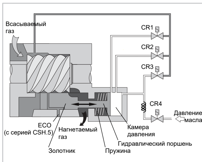
Рис. 8: Гидравлическая схема для двойного регулирования производительности с CR золотником и соленоидными клапанами CR1 .. 4. (У компрессоров CSW и CSH.6 порт ECO встроен непосредственно в корпус.)
