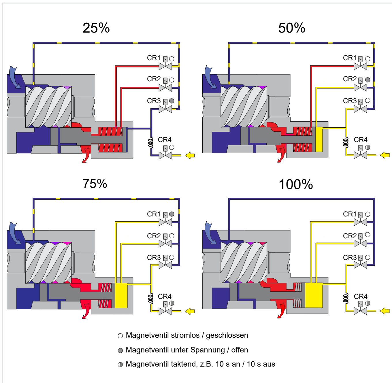
Abb. 9: Stufige Leistungsregelung mit CR-Schieber, 25 .. 100%.
