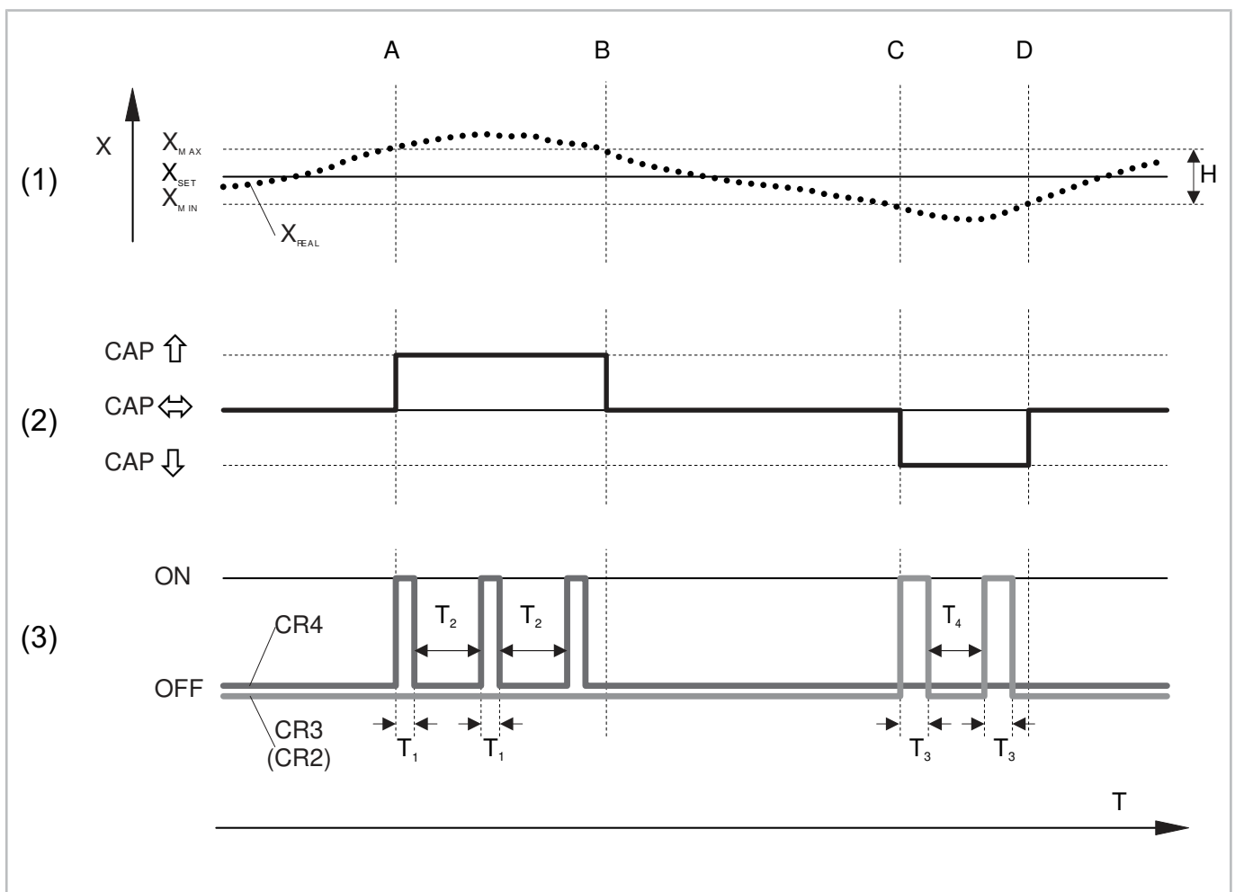
Abb. 10: Stufenlose Leistungsregelung
