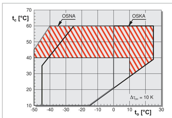
Abb. 14: Einsatzgrenze OS.A95 und OS.A105 Schraubenverdichter bei ECO-Betrieb. Im schraffierten Bereich ist das ECO Dämpfersystem vorgeschrieben.
