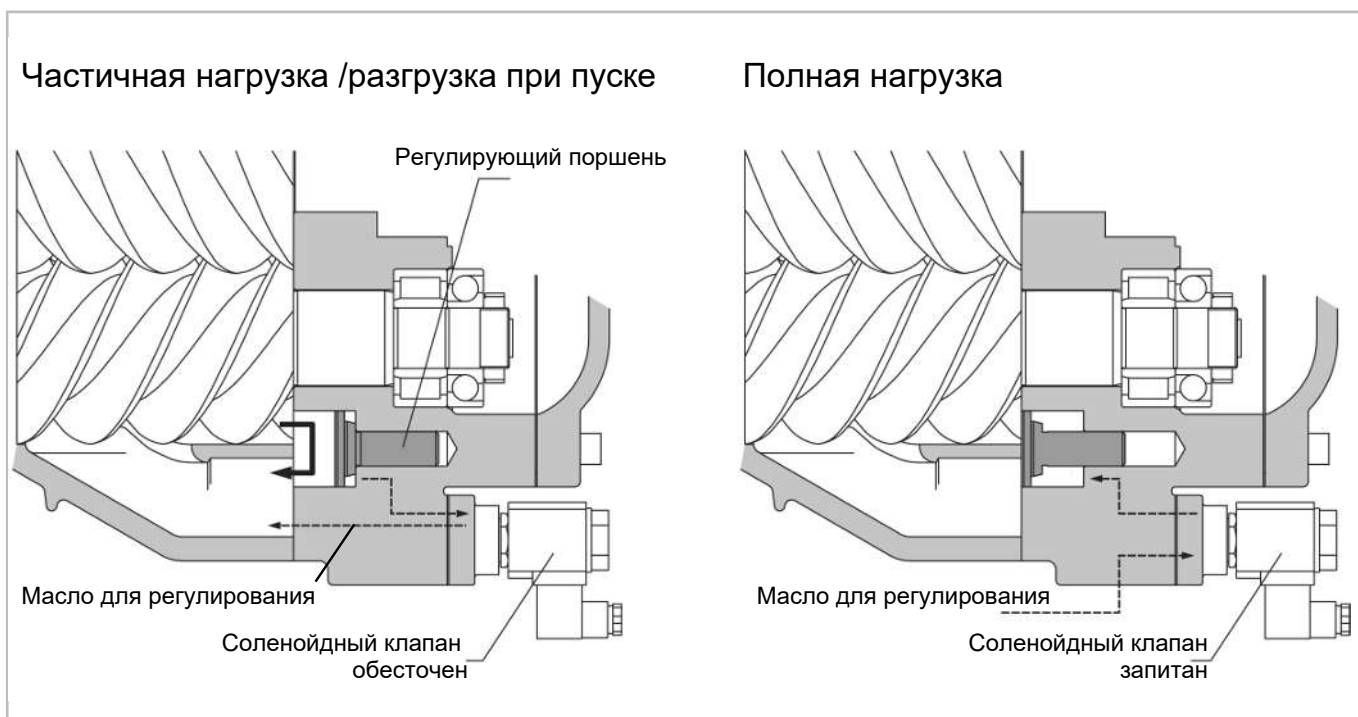
Рис. 3: Конструкция регулятора производительности или разгрузки при пуске компрессоров OS.74. На рисунке показан один из двух регулирующих поршней и соответствующий солёный клапан. Для компрессоров OS.53 и OS.7441 принцип работы аналогичен, но перепускной канал на сторону всасывания расположен на периферии ведущего ротора.
